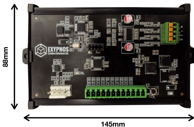
DIN Rail
